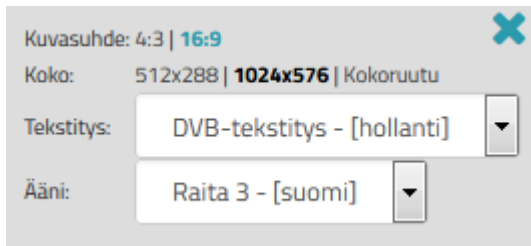
Kuva 5.2. Tekstityskielen valinta
