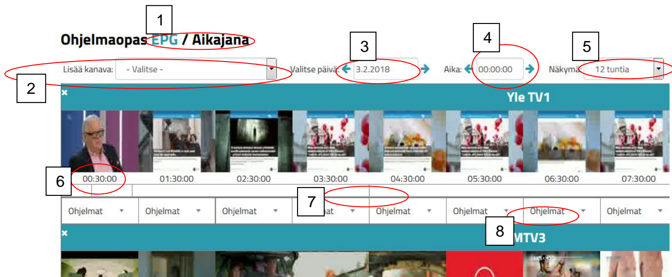
Kuva 3.4 Aikajananäkymä
