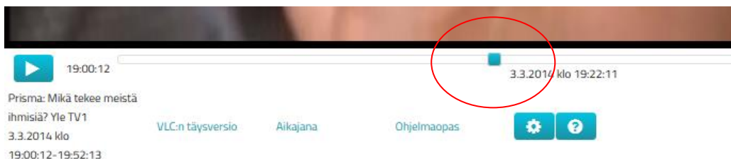
Kuva 5.1 Kohdistin
