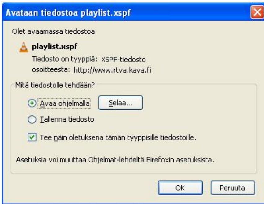
Kuva 5.5 Avataan tiedostoa...
