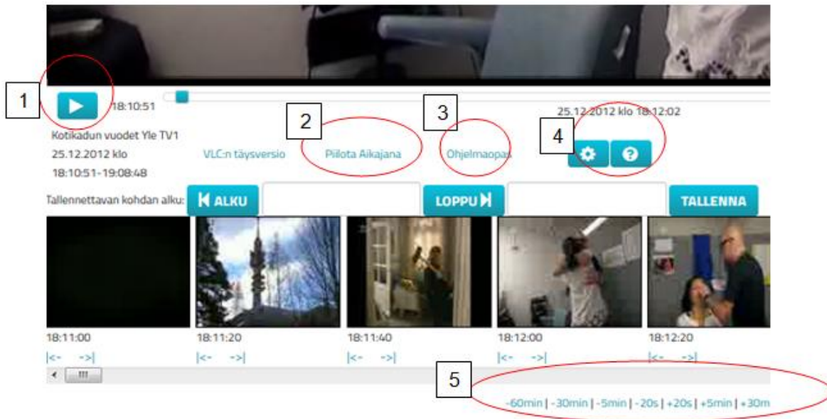
Kuva 5.4 VLC:n navigointi
